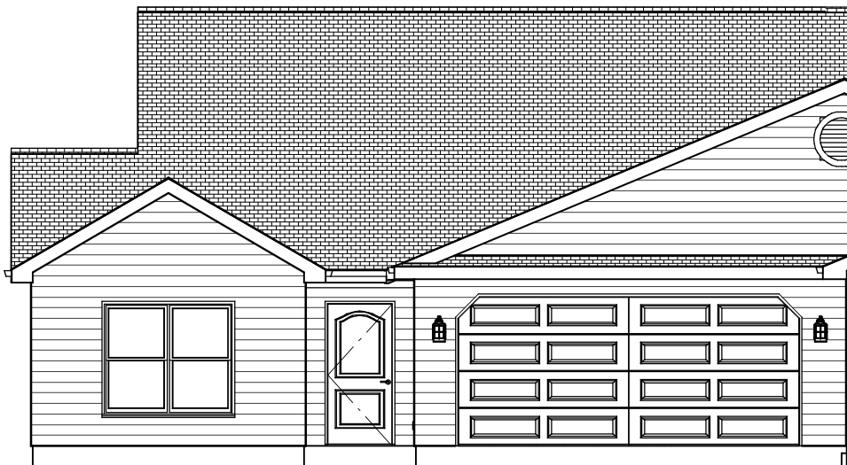
Elevation B
