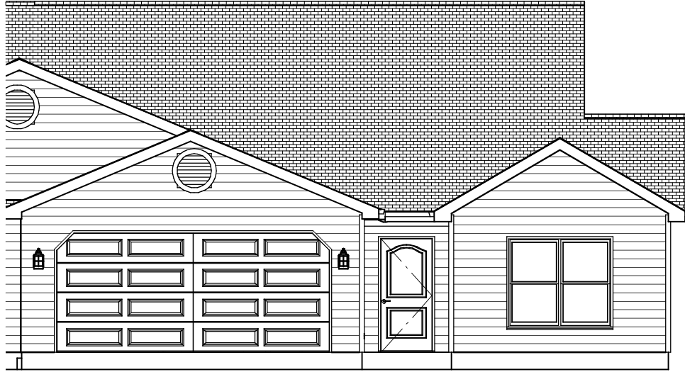
Elevation A
